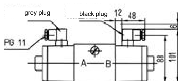
Z4 angled plug
